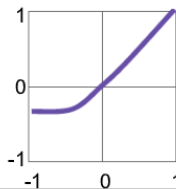
Exponential LU
