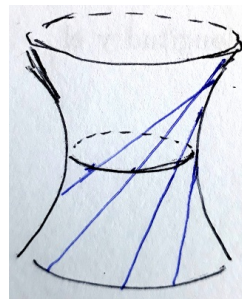
Catenoide
